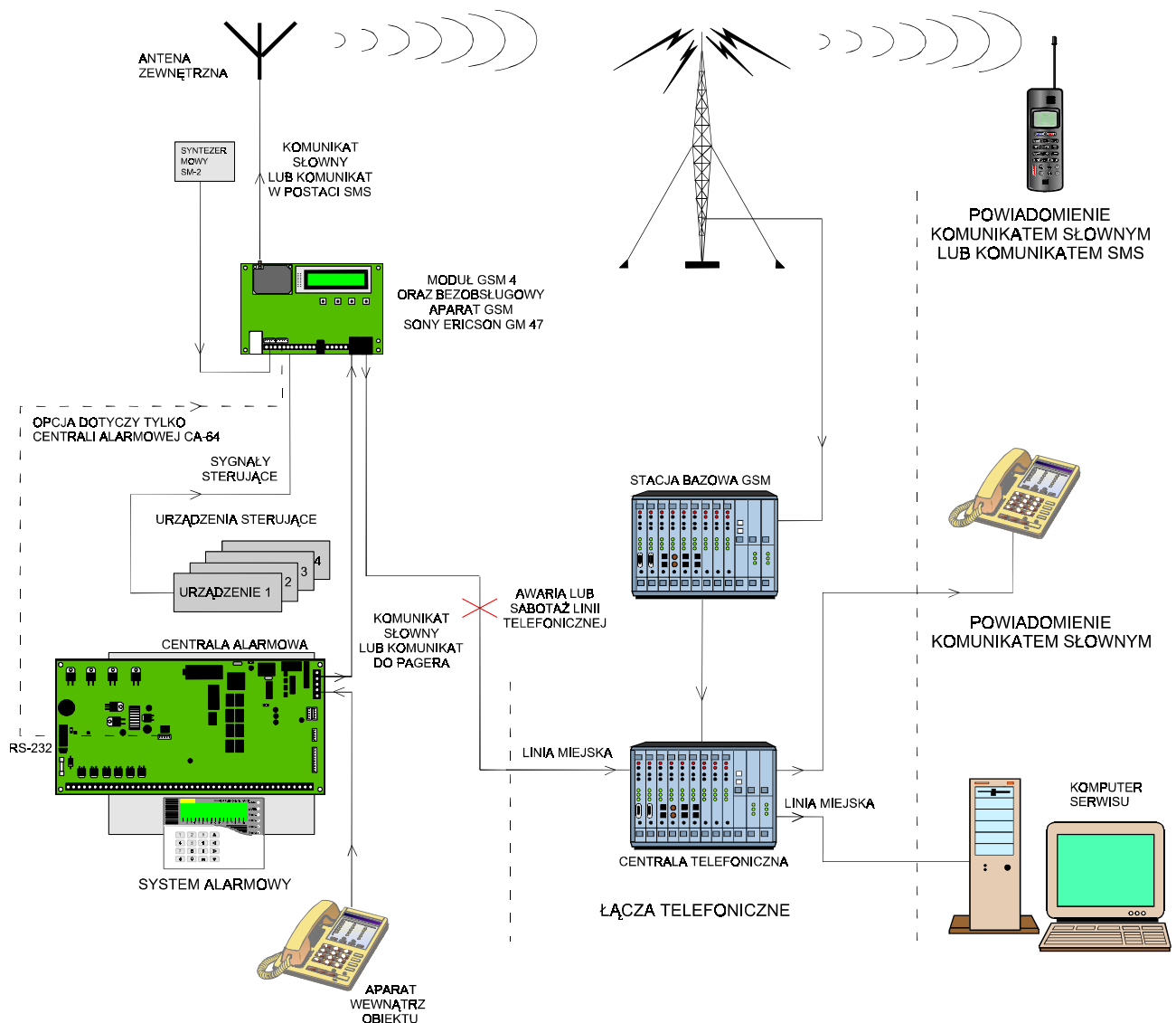
Rysunek 1. Sposób włączenia modułu w linię telefoniczną - strzałki wskazują sposób powiadomienia o alarmie w przypadku uszkodzenia lub braku linii telefonicznej.
