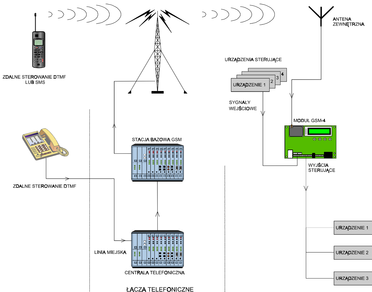
Rysunek 8. Sposób realizacji zdalnego sterowania stanem wyjść i blokadą wejść modułu.
